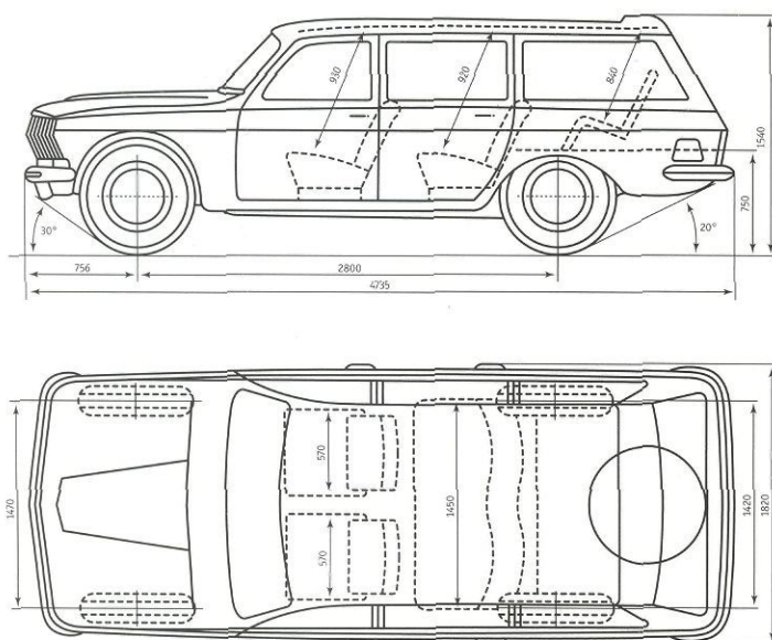
Схема автомобиля ГАЗ-24-02 «Волга»
